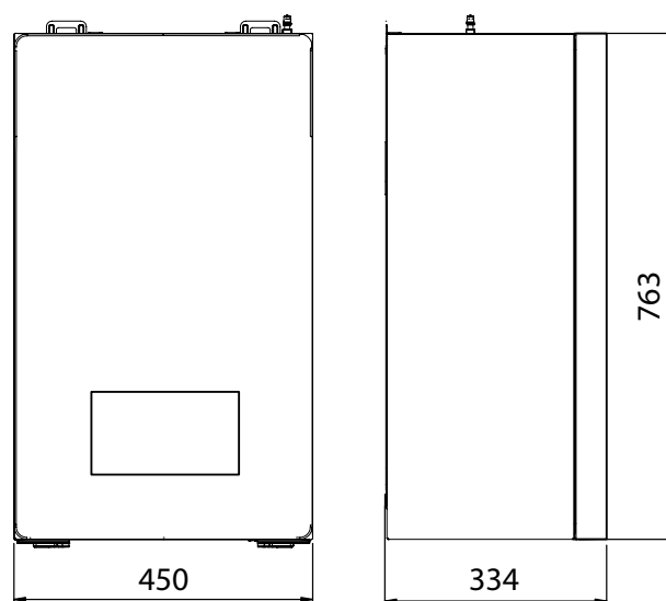
Dimensiuni de gabarit
